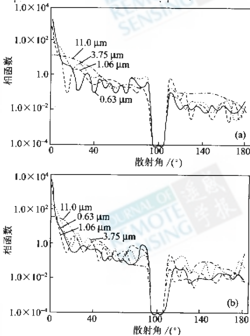
图 1 球形沙尘粒子在不同波长的 Mie 散射相函数曲线
